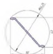
Алюминиевый профиль Р 129, вес 0,285 кг/п.м. (лопасть облегченная для решёток АНР)
