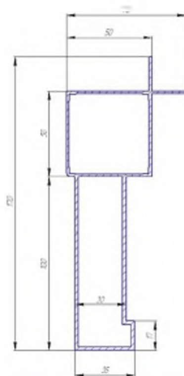
Алюминиевый профиль P 151-45 BAS, вес 2,295 кг/п.м.
