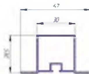
Алюминиевый профиль P 231-25, вес 0,691 кг/п.м.
