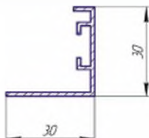
Алюминиевый профиль НЧП 5297 (рамка решёток АМН), вес 0,242 кг/п.м.
