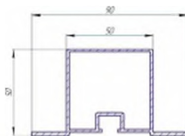
Алюминиевый профиль P 250-45, вес 1,158 кг/п.м.
