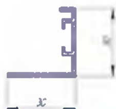
Алюминиевый профиль NCH 5297 (рамка решёток АМН)
