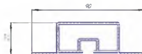
Алюминиевый профиль P 250-25, вес 1,156 кг/п.м.
