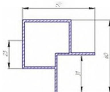
Алюминиевый профиль Р 140-25000, вес 0,734 кг/п.м.
