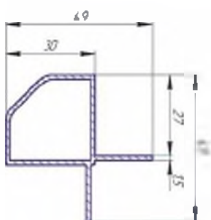
Алюминиевый профиль S 1300-25, вес 0,586кг/п.м
