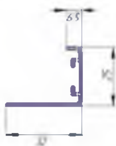
Алюминиевый профиль НЧП 3072 (рамка решеток АЛН, АНР), Вес 0,168 кг/п.м
