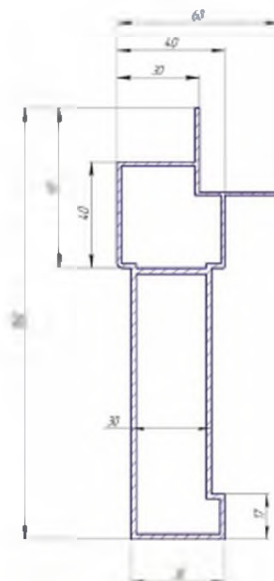
Алюминиевый профиль BAS 140-250, вес 2,187 кг/п.м.
