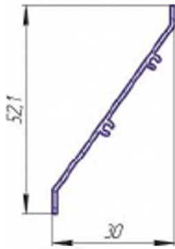
Алюминиевый профиль АП 258 (жалюзи решеток АНР), вес 0,211 кг/п.м
