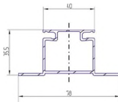
Алюминиевый прсфиль НЧП 4415, вес 0,852 кг/п.м
