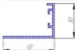
Алюминиевый профиль НЧП 755 (рамка решеток АЭН, АМР)
