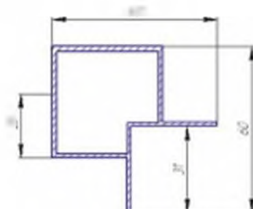
Алюминиевый профиль P 140-25, вес 0,734 кг/п.м
