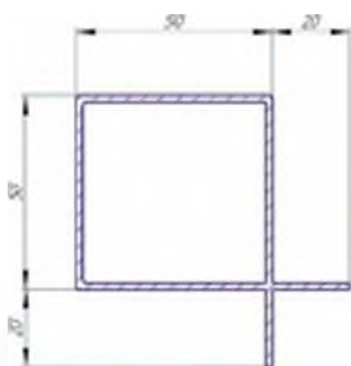
Алюминиевый профиль P 150-45, вес 1,023 кг/п.м.
