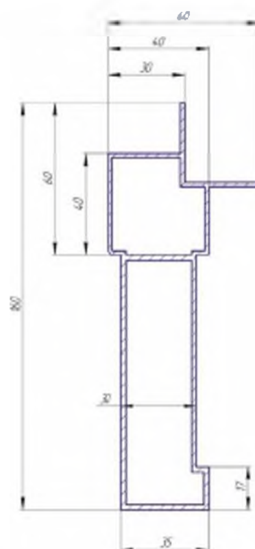
Алюминиевый профиль P 140-25 BAS, вес 2,187 кг/п.м.
