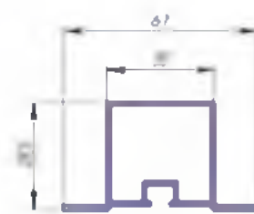
Алюминиевый профиль P 231-25000, вес 0,691 кг/п.м.
