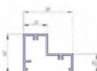
Р 121 алюминиевый профиль. (рамка для решеток АНР)
