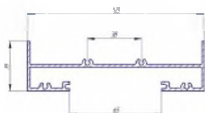
Алюминиевый профиль PS 120, вес 1,574 кг/п.м. (боковина для клапана АВК)
