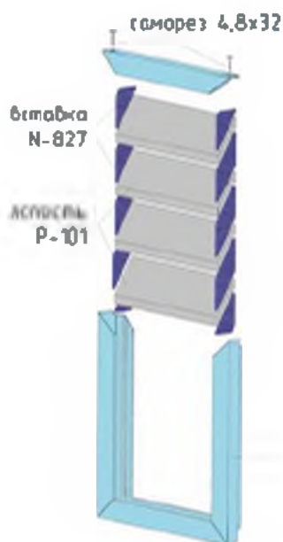
Схемы сборки решёток
