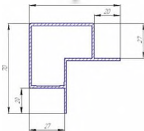
Алюминиевый профиль P 150-25, вес 1,253 кг/п.м.
