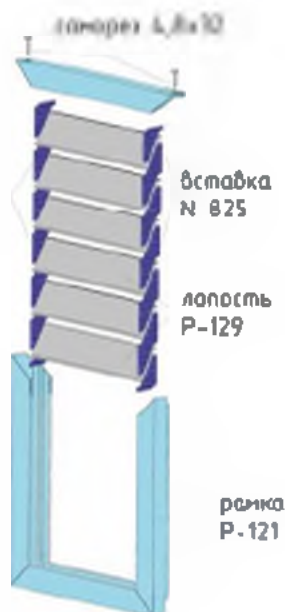
Схемы сборки решёток
