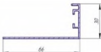
Алюминиевый профиль НЧП 5298 (рамка решёток АДР)
