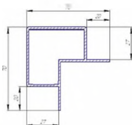
Алюминиевый профиль P 150-25000, вес 1,253 кг/п.м
