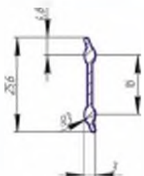
Алюминиевый профиль НЧП 5299 (лицевая часть клапана АМР, АДР)
