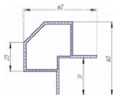
Алюминиевый профиль S 1400-25, вес 0,894 кг/п.м
