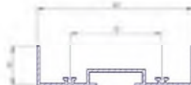
Алюминиевый профиль P 125, (боковина ражки клапана АВК)
