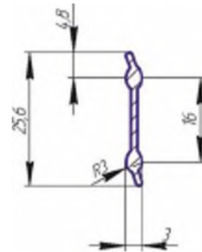
Алюминиевый профиль НЧП 5299 (лопость клапана АНР, АДР), вес 0,112 кг/п.м.
