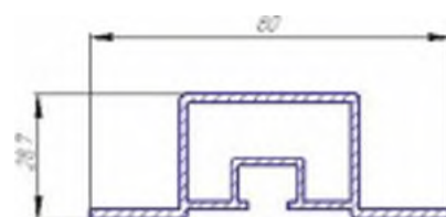
Алюминиевый профиль P 240-25, вес 1,807 кг/п.м.
